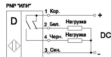
Рисунок 2 - Схема подключения
